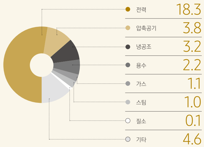
유형별 에너지 비용 절감
