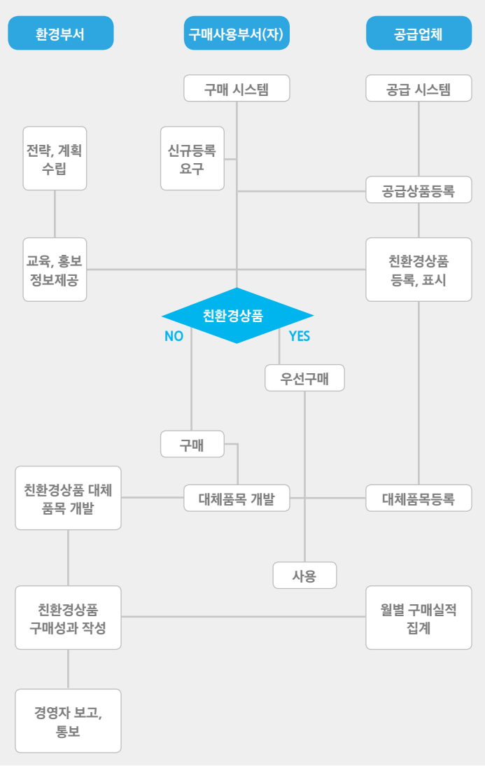
녹색구매 프로세스
