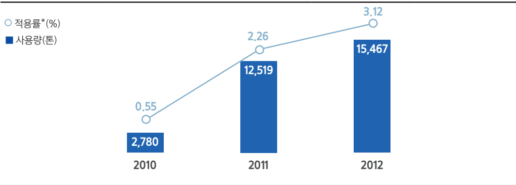
재생플라스틱 사용량
